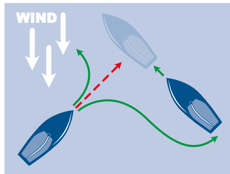
Abbildung 6 Ausweichen Segelfahrzeuge untereinander mit dem Wind nicht von derselben Seite, Regel 12 (a) (i) der KVR
